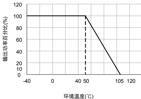
环境温度降额曲线图
