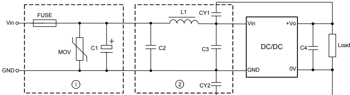
图2 EMC 推荐应用电路
