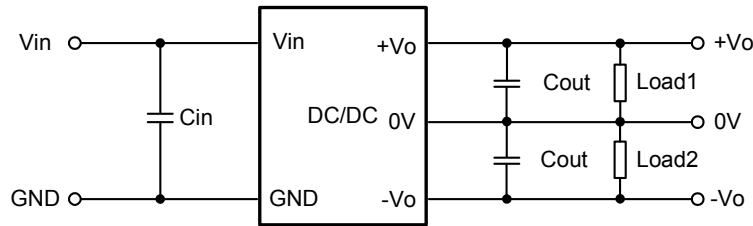
图1 一般推荐应用电路
