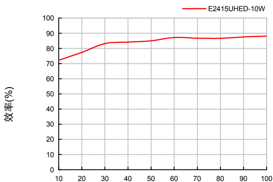
效率与负载关系曲线图 (标称电压输入)
