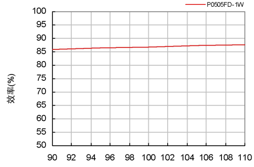
效率与输入电压关系曲线图(满载)
