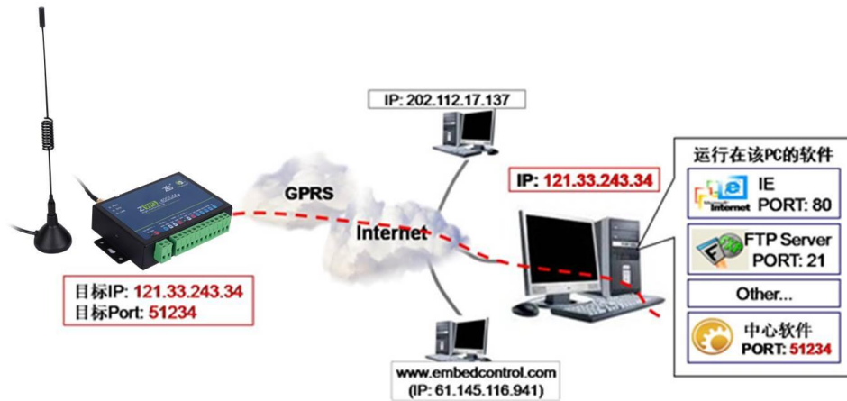
图 3.1 IP 地址及端口号的用途
