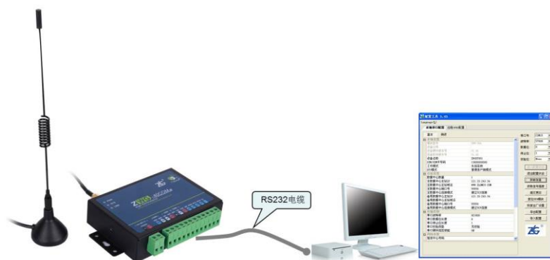
图 3.3 本地配置示意图
