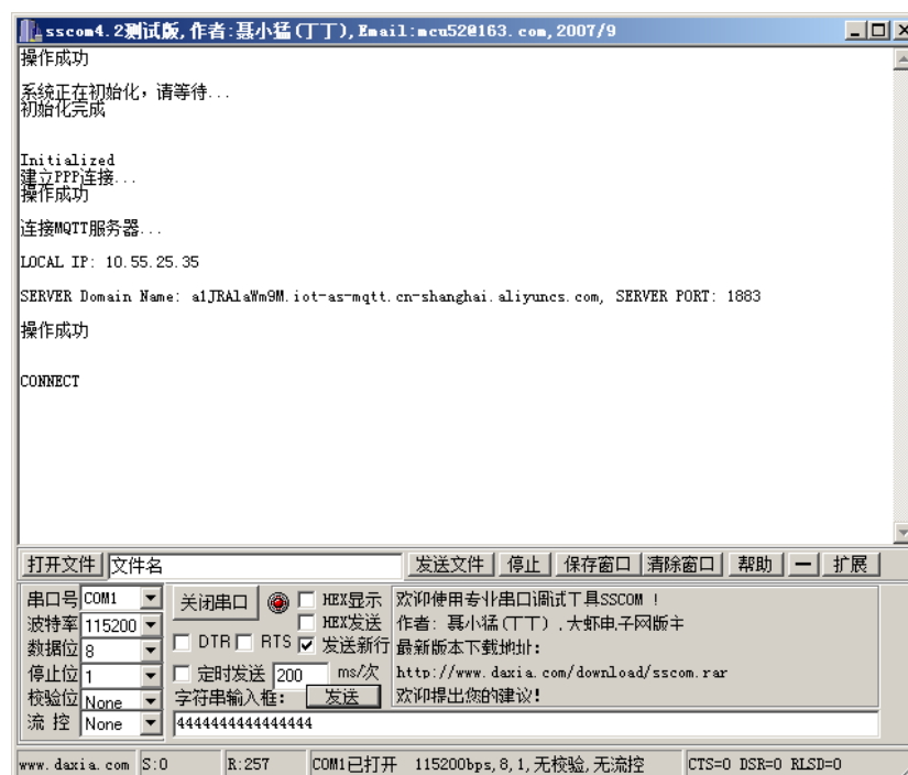
图 4.6 与标准 MQTT 服务器建立连接
