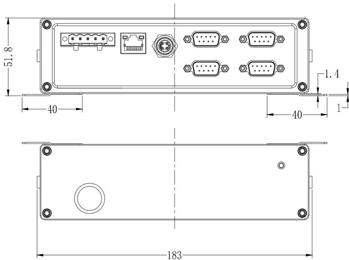
图 3.3 主机尺寸图三
