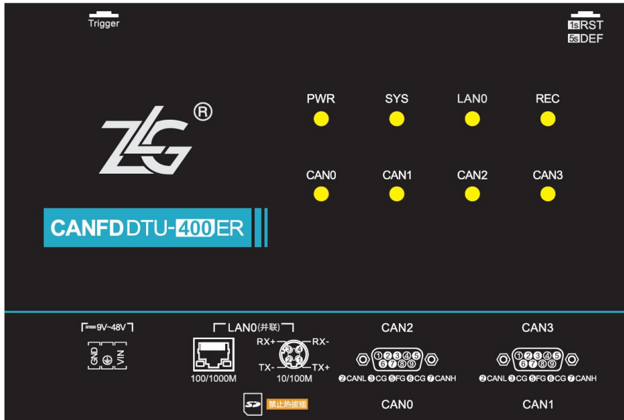
图 4.1 面板布局
