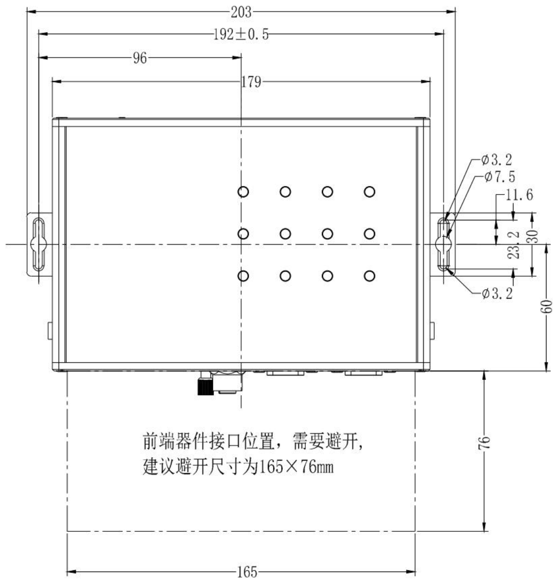
图 3.1 主机尺寸图一
