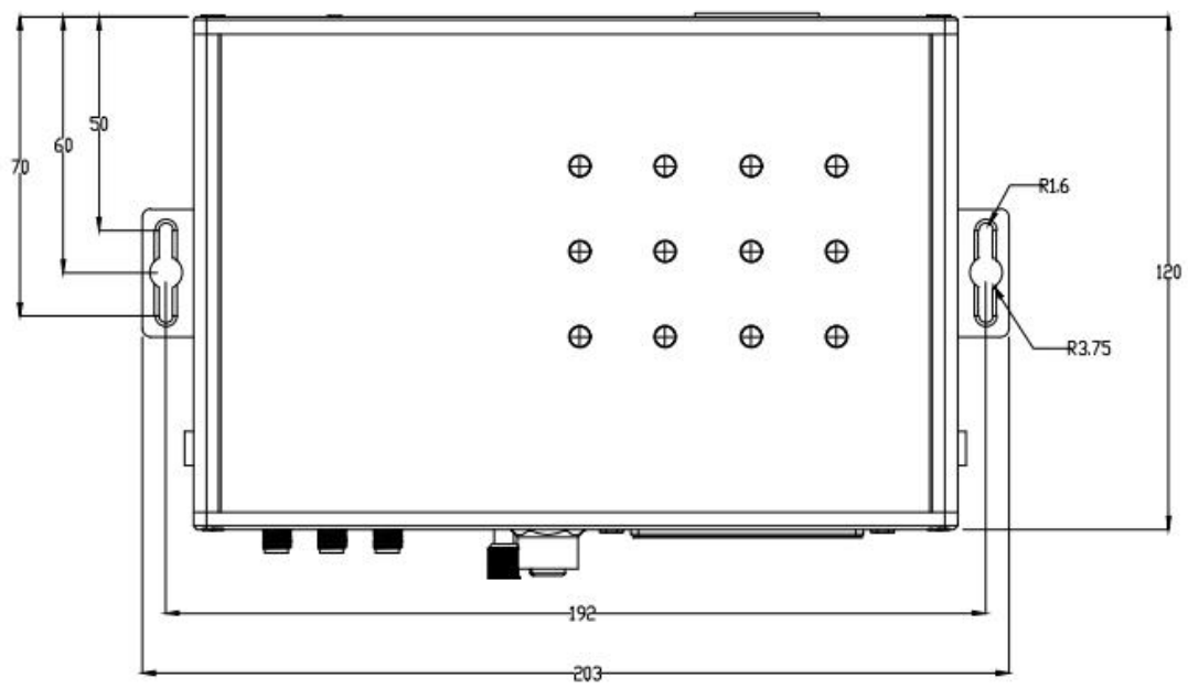
图 4 主机尺寸图三
