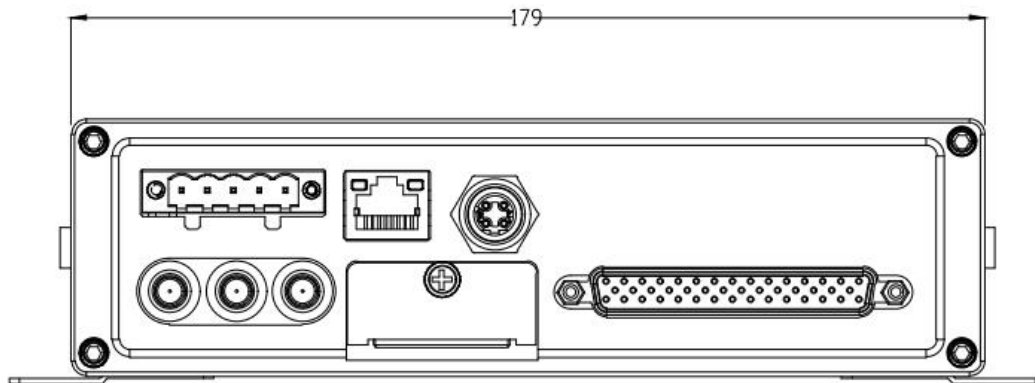
图 2 主机尺寸图一
