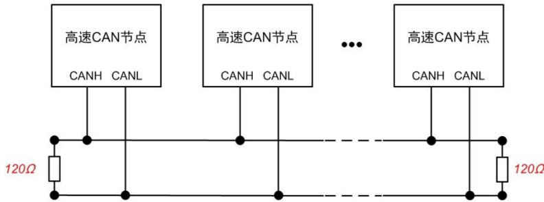
图 6 高速 CANFD 典型网络连接示意图
