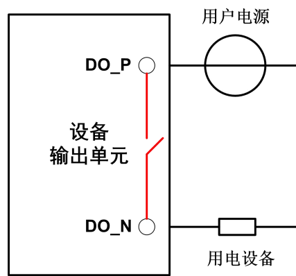
图 8 DO 网络连接示意图
