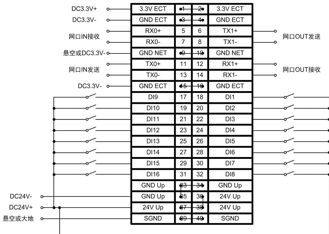
图 4.2 ZIOC-E1600DP 典型接线图
