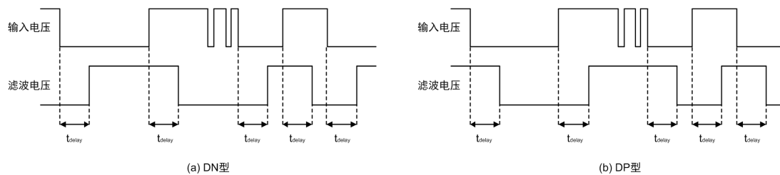
图 6.1 消抖滤波
