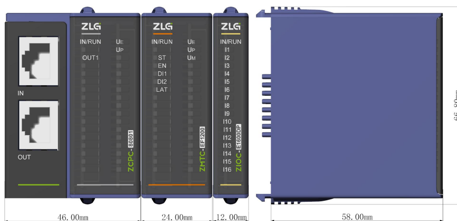
图 3.1 尺寸图
