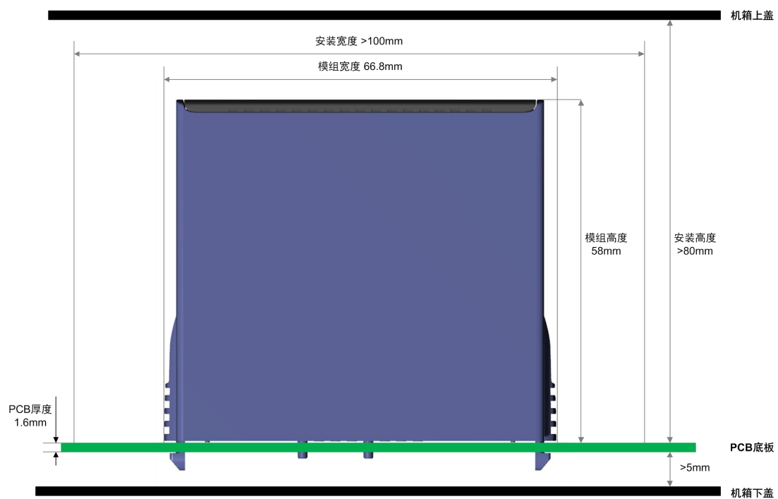
图 3.3 安全距离
