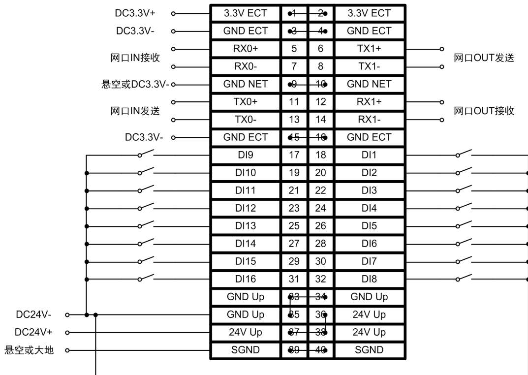
图 4.1 ZIOC-E1600DN 典型接线图
